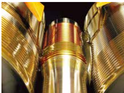
ボルトの転造加工(最大M300まで)
